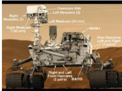
Vehículo explorador tipo rover: Curiosity
